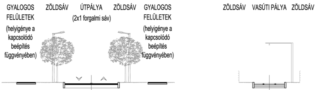
3.A - 3.A Egyvágányú vasúti pálya
